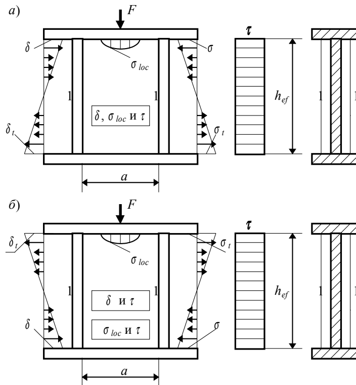
Рис. 12. Схема балки, укрепленной поперечными основными ребрами жесткости (1) a – сосредоточенная нагрузка F приложена к сжатому поясу; б – то же, к растянутому поясу
