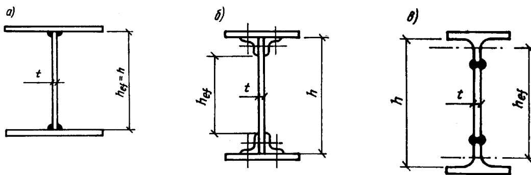
Рис. 10. Расчетная высота стенки составной балки а – сварной из листов; б – на высокопрочных болтах; в – сварной с таврами
