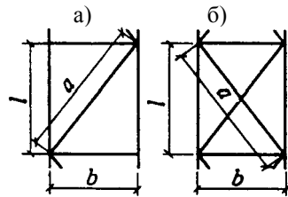
Черт. 3. Схема решетки
