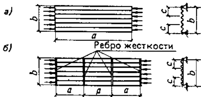
Черт. 12. Расчетная схема сжатого гофрированного листа
