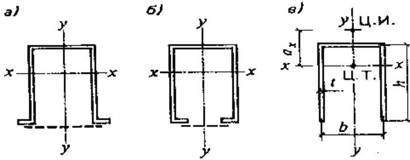
Черт. 2. П-образные сечения элементов а,б — усиленные планками или решеткой; в — открытое
